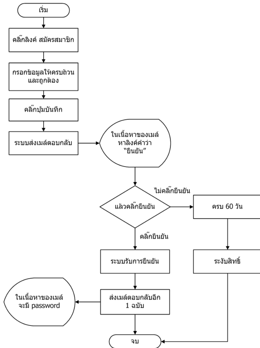
รูปที่ 5. แสดงลำดับขั้นตอนการสมัครสมาชิก
